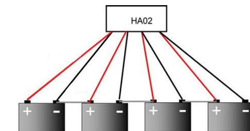
Rys.1. Podłączenie stabilizatora w akumulatorach połączonych w szereg
