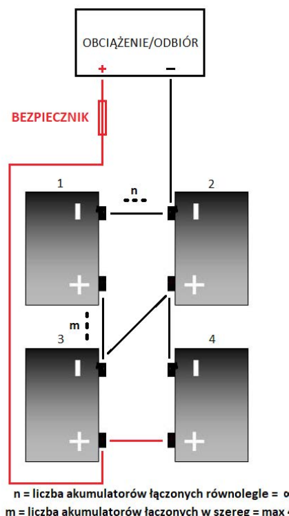
Rys.4. Schemat szeregowo-równoległego połączenia akumulatorów
