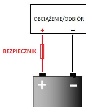
Rys.1. Schemat podłączenia pojedynczego akumulatora
