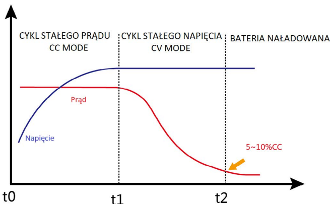
Rys.1. Metoda ładowania ładowarkami Kon-TEC z serii DL.
